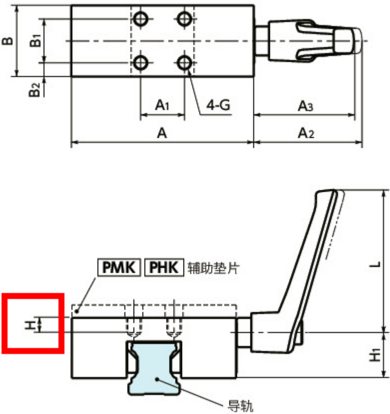
HK 形状图
