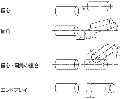
図2 ミスアライメントの種類
