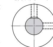
図1 Dカット軸とハブの位置
