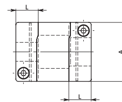
クランピングタイプ XGT2-C XGS2-C XGL2-C
