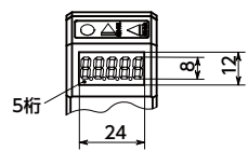
ディスプレイ部詳細
