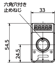
六角穴付き 止めねじ
