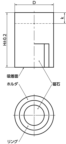
JST-AN-TZB アルニコ・外径公差D ±0.2
